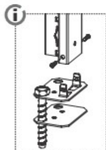
Bodenverankerung Set mit Bodenanker und Blechblechbohrer (Art.-Nr. 12709)
